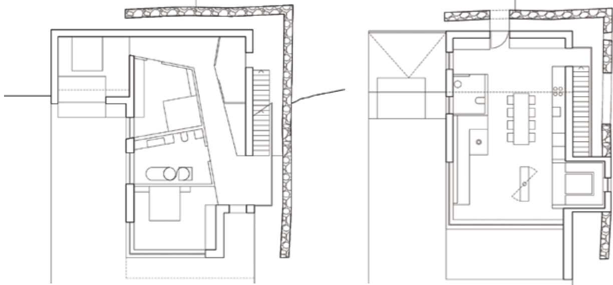
Grundriss Erdgeschoß
