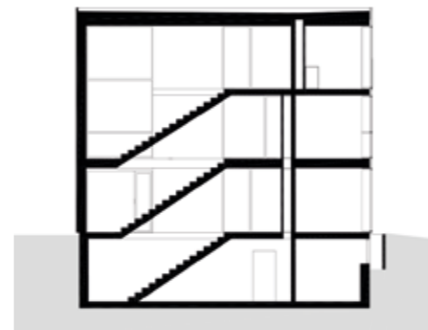
Schnitte
