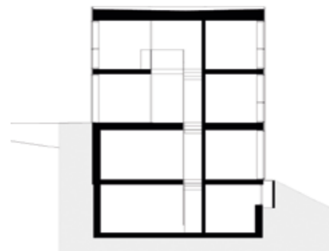
Schnitte
