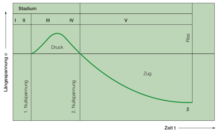
b. Betonspannungen bei behinderter Verformung
