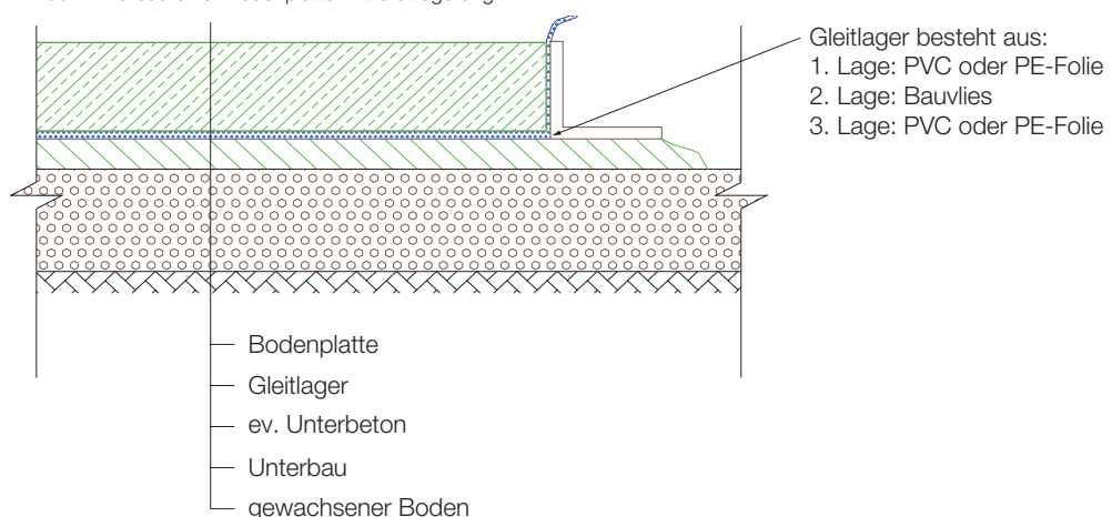
Abb. 2: Aufbau einer Bodenplatte mit Gleitlagerung
