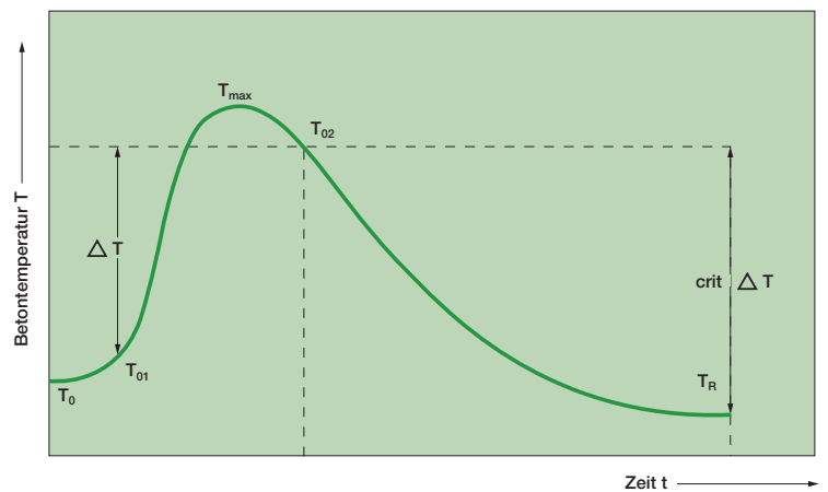
Abb. 1: Verhalten des Betons während der Erhärtung
